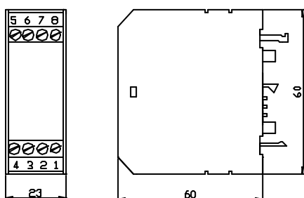
23 mm-DIN-rail module
