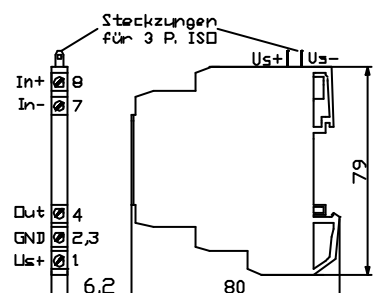
6.2 mm DIN-rail-module
